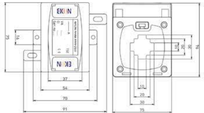
EK30D-AKIM TRAFOLARI
