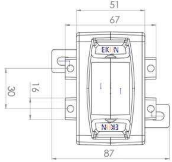
EK60DR-AKIM TRAFOLARI
