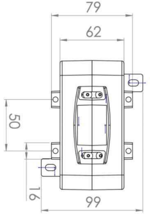
EK100DR-AKIM TRAFOLARI
