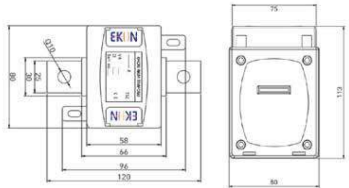
EK30-AKIM TRAFOLARI
