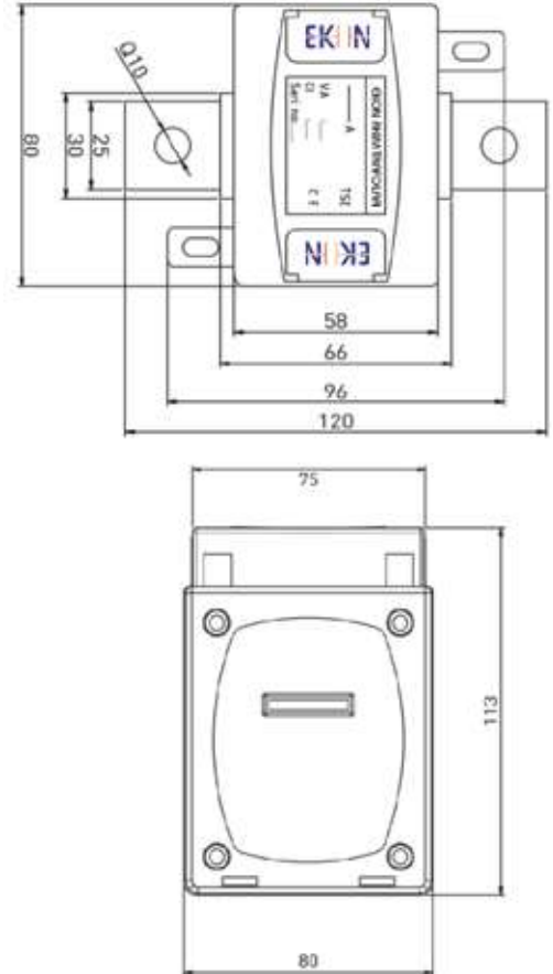
EKB-AKIM TRAFOLARI
